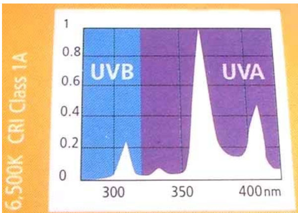
Spettro sulla confezione
